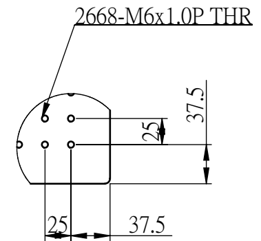
細部放大圖 A 比例 1:5
