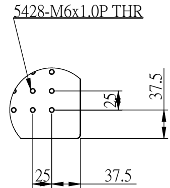
細部放大圖 A 比例 1:5
