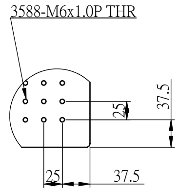
細部放大圖 A 比例 1:5
