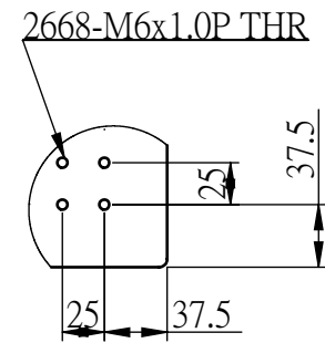
細部放大圖 A 比例 1 : 5
