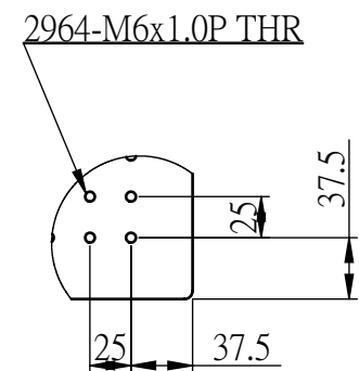
細部放大圖 A 比例 1:5
