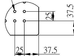
細部放大圖 A 比例 1 : 5
