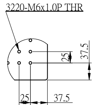
細部放大圖 A 比例 1:5
