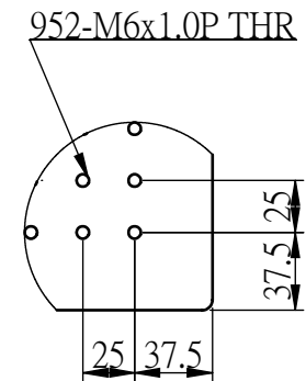
細部放大圖 A 比例 1:4
