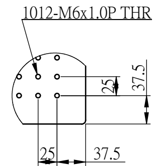
細部放大圖 A 比例 1 : 5
