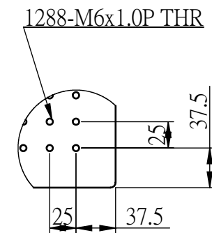
細部放大圖 B 比例 1:5
