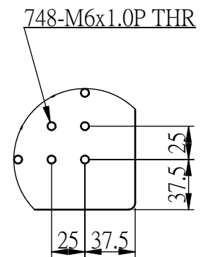
細部放大圖 A 比例 1:4
