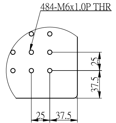
細部放大圖 A 比例 1:3
