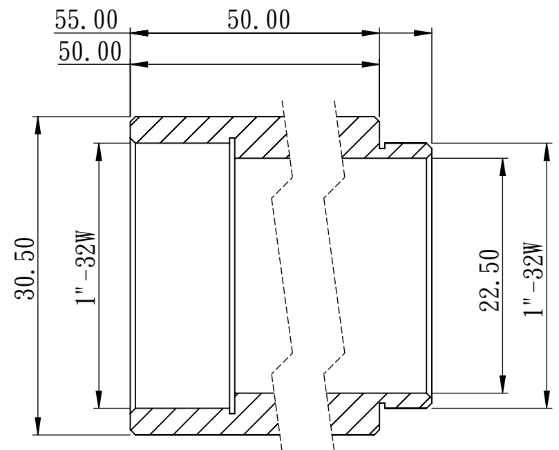
剖面圖 A-A
