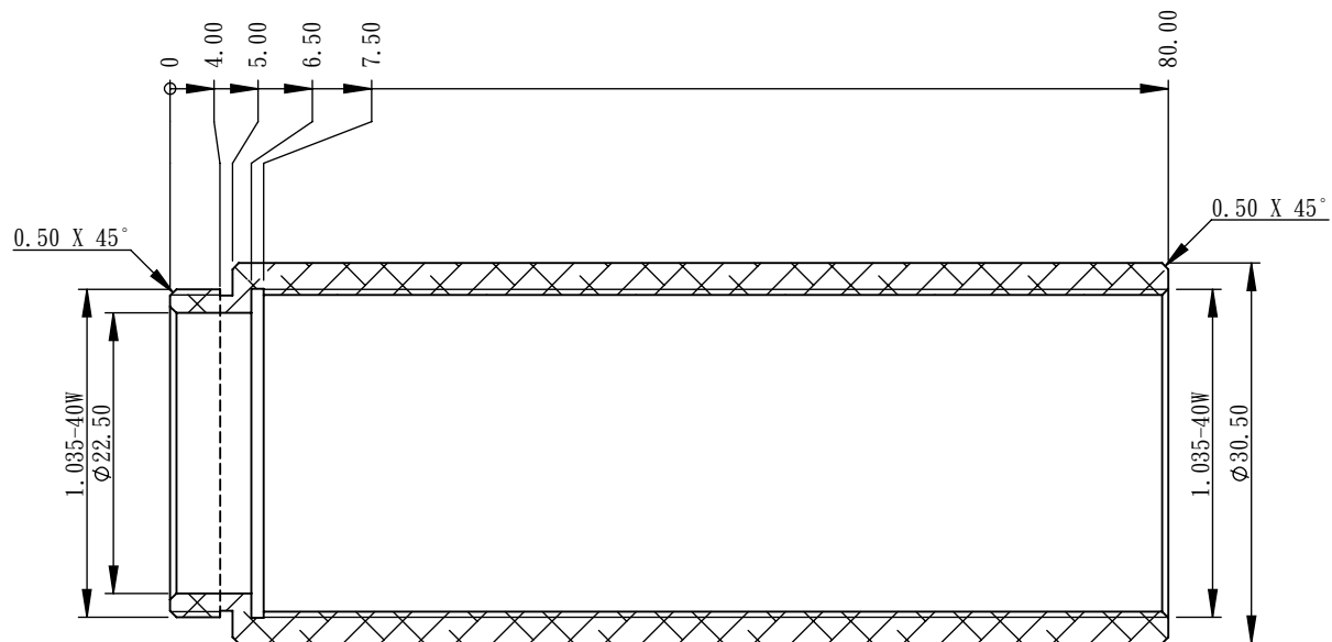
剖面圖 A-A 比例 3 : 2
