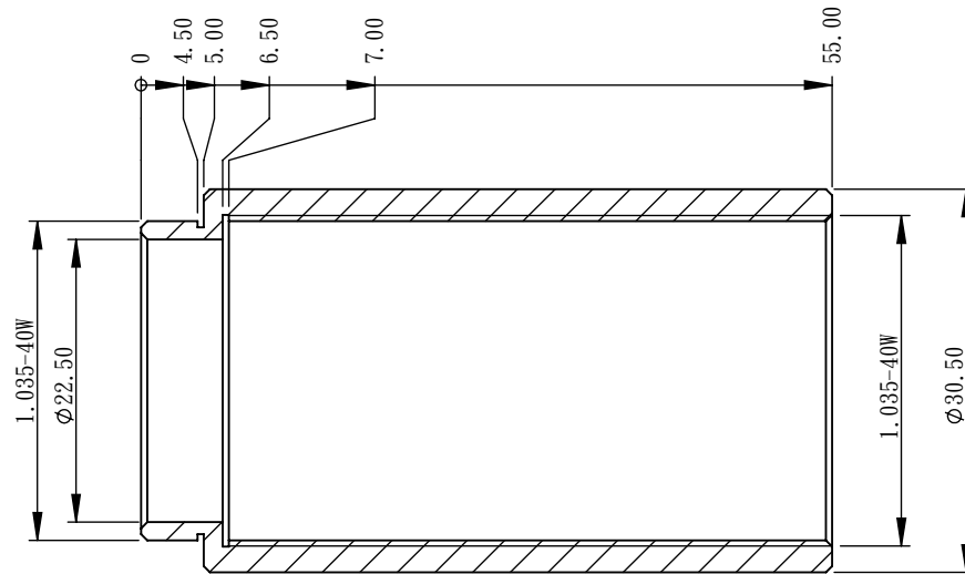
剖面圖 A-A 比例 3 : 2
