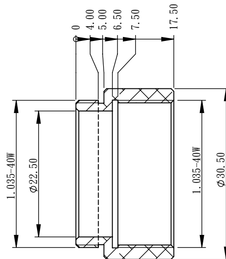
剖面圖 A-A 比例 3 : 2
