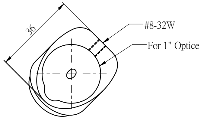
視圖 A
